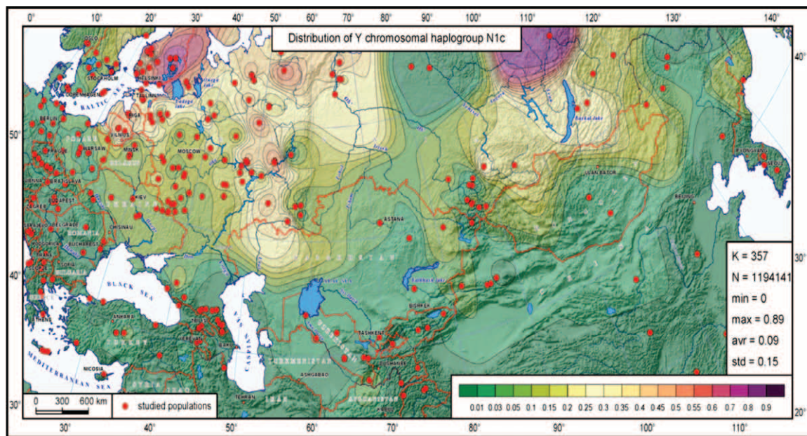
Рис. 1. Карта распространения гаплогруппы N1c 1 .
