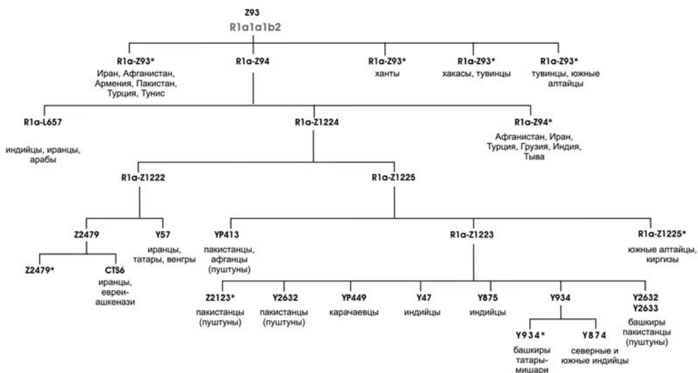
Схема 2. Филогенетическое древо субклада R1a1-Z93.
