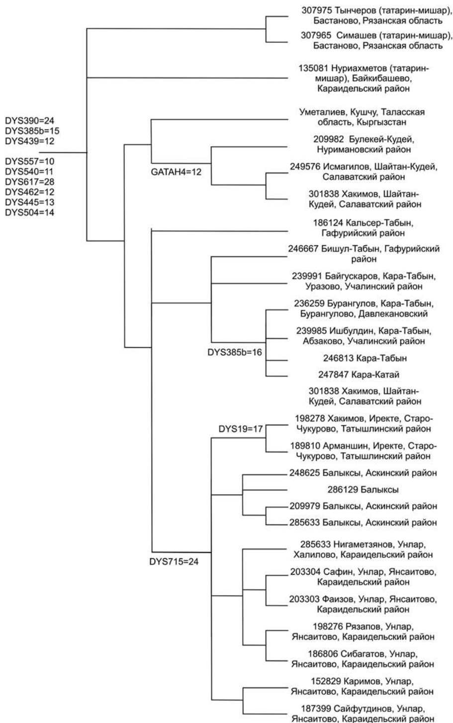
Схема 1. Филогенетическое древо «Майкыбиевичей».
