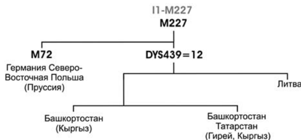
Рис. 2. Филогенетическое древо
